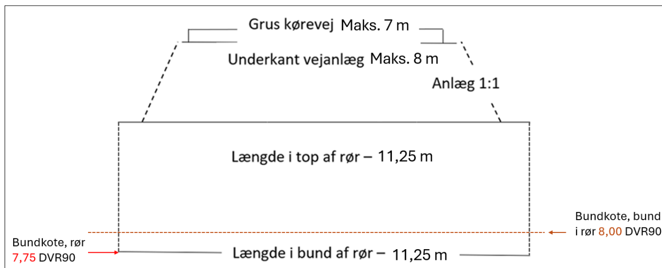
Figur 2. Principskitse for røroverkørslen med angivelse af anlæg og koter.
